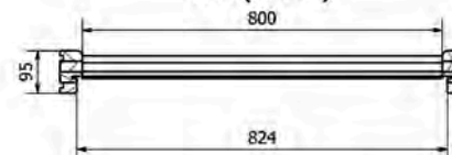
A-A (1 : 8)
