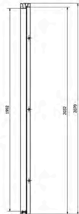
B-B (1 : 8)
